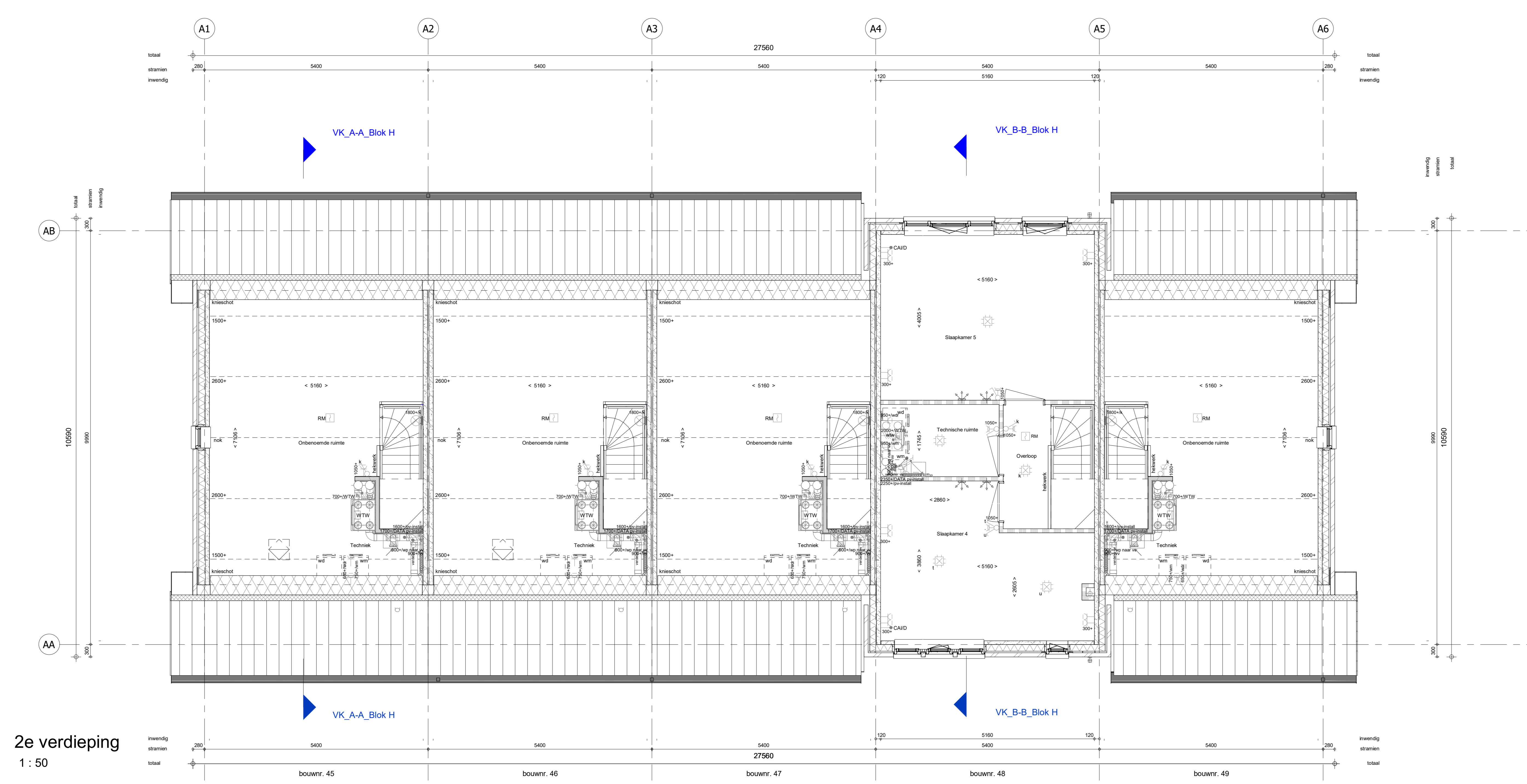
dakplan 1 : 50
